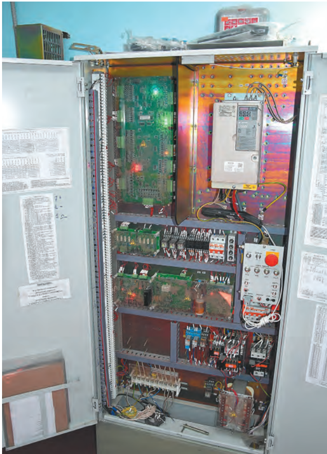
Начинка современного лифтового оборудования
