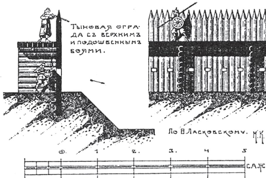
Строение тыновой ограды Егошихинской крепости
